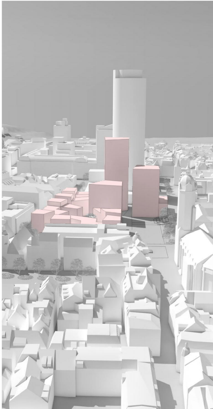
drei Hochpunkte
