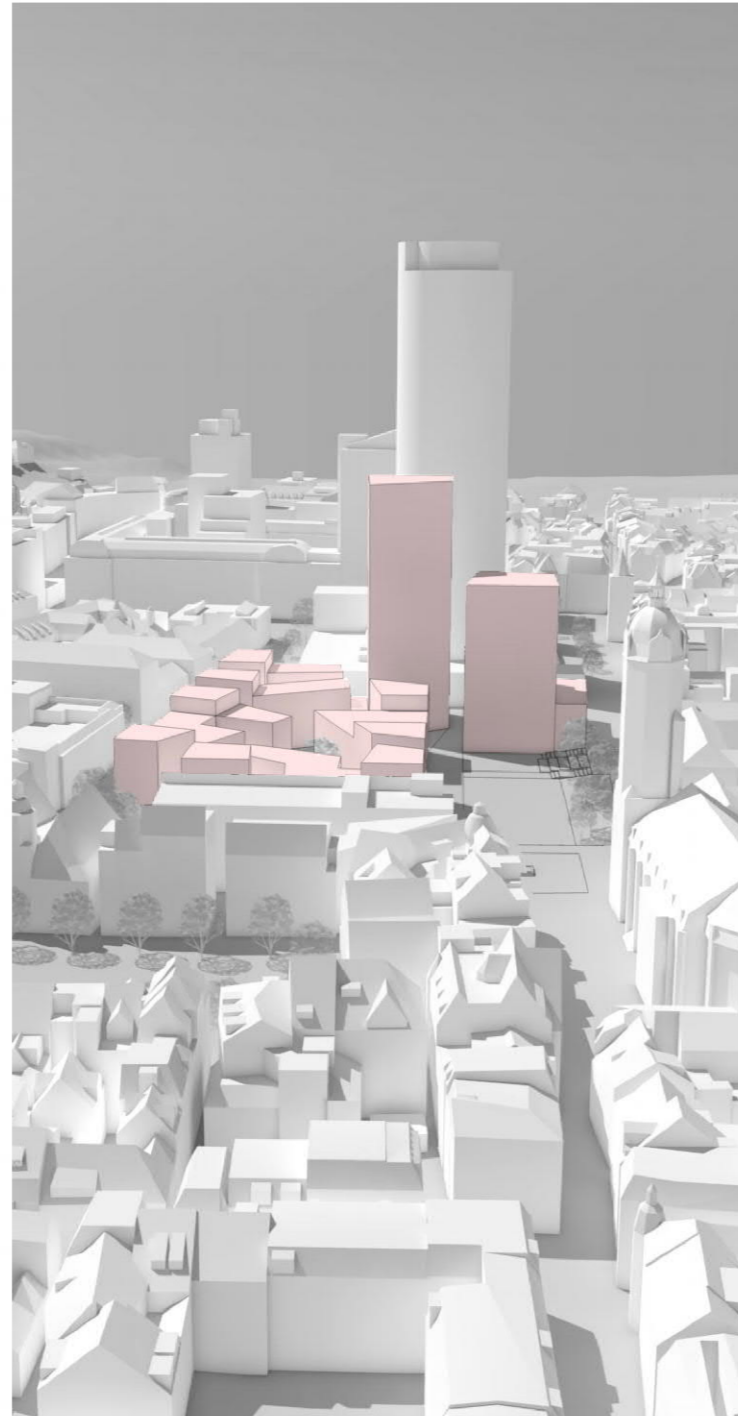
zwei Hochpunkte
