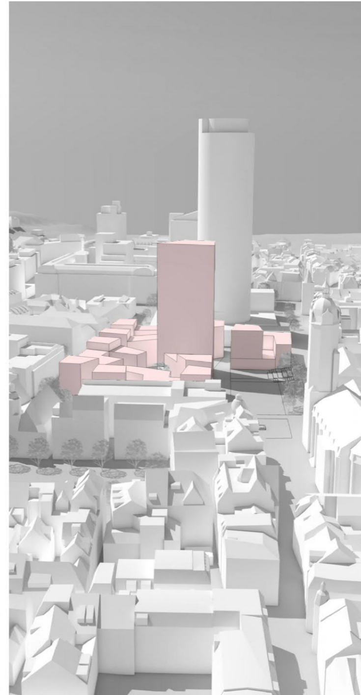
ein Hochpunkt
