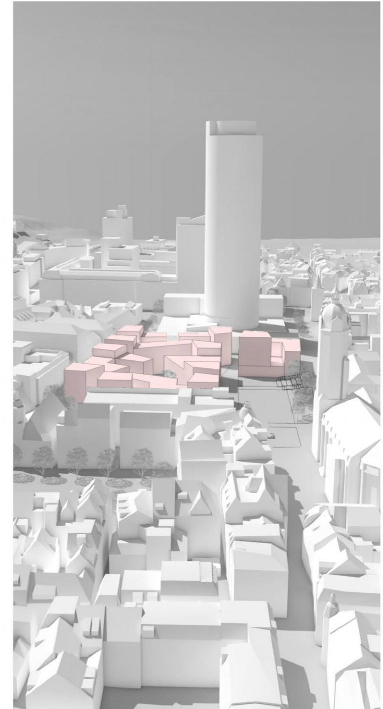
kein Hochpunkt
